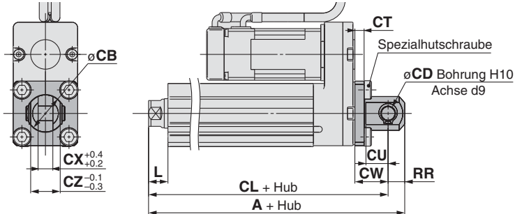
Gabelbefestigung: LEY16□□B-□□□D
