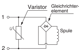
ohne Betriebsanzeige
