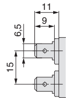
Abmessungen der Klemmen beim Flachstecker Serie 250
