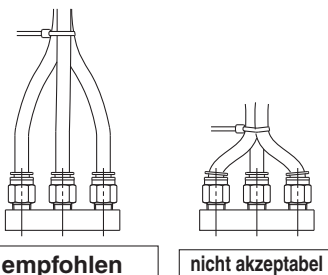
Abb. 2 Schlauchverbindung mit Kabelbinder
