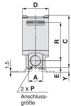
Abmessungen der Klemmen beim Flachstecker Serie 250
