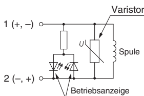
mit Betriebsanzeige/Funkenlöschung
