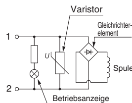
mit Betriebsanzeige
