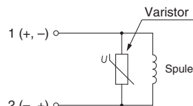
mit Funkenlöschung
