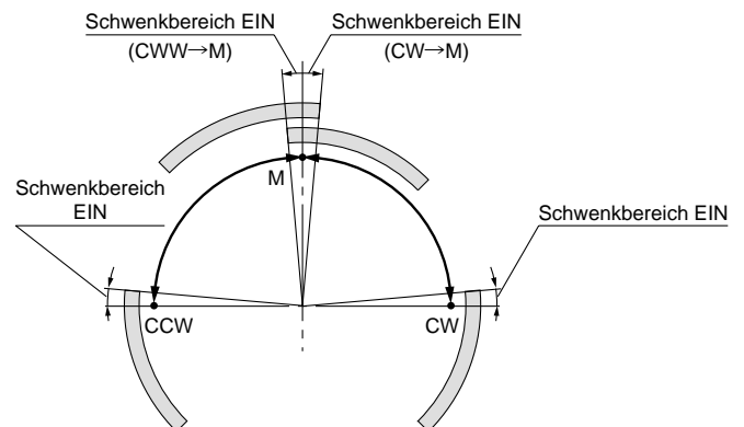
Signalgeber zur Abfrage der Mittelstellung: 2 Stk.
