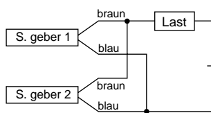
2-Draht-System mit 2 parallel geschalteten Signalgebern (OR)
