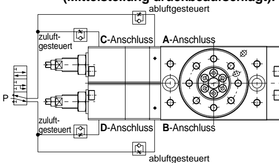
Abb. 1 5/3-Wege-Elektromagnetventil (Mittelstellung druckbeaufschlagt): 1 Stk.
