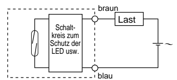
2-Draht-System <Reedkontakt-Signalgeber>
