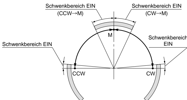
Signalgeber zur Abfrage der Mittelstellung: 1 Stk.
