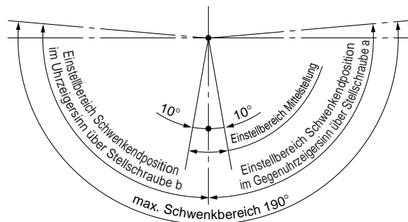
Abb. 5 Winkeleinstellbereich
