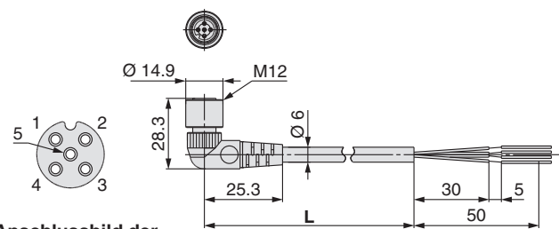
Anschlussbild der Buchse A-codiert
